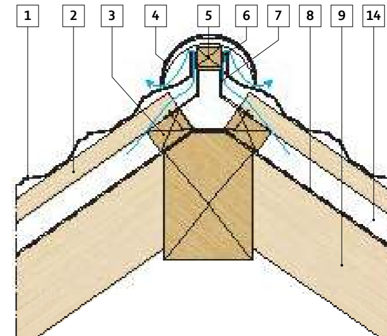
Вариант 1: Схема в разрезе
