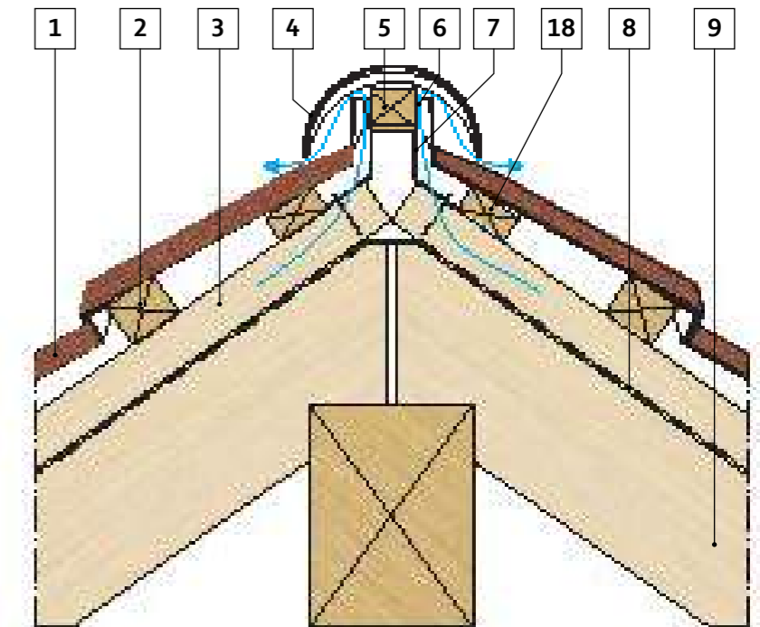
Вариант 1: Схема в разрезе
